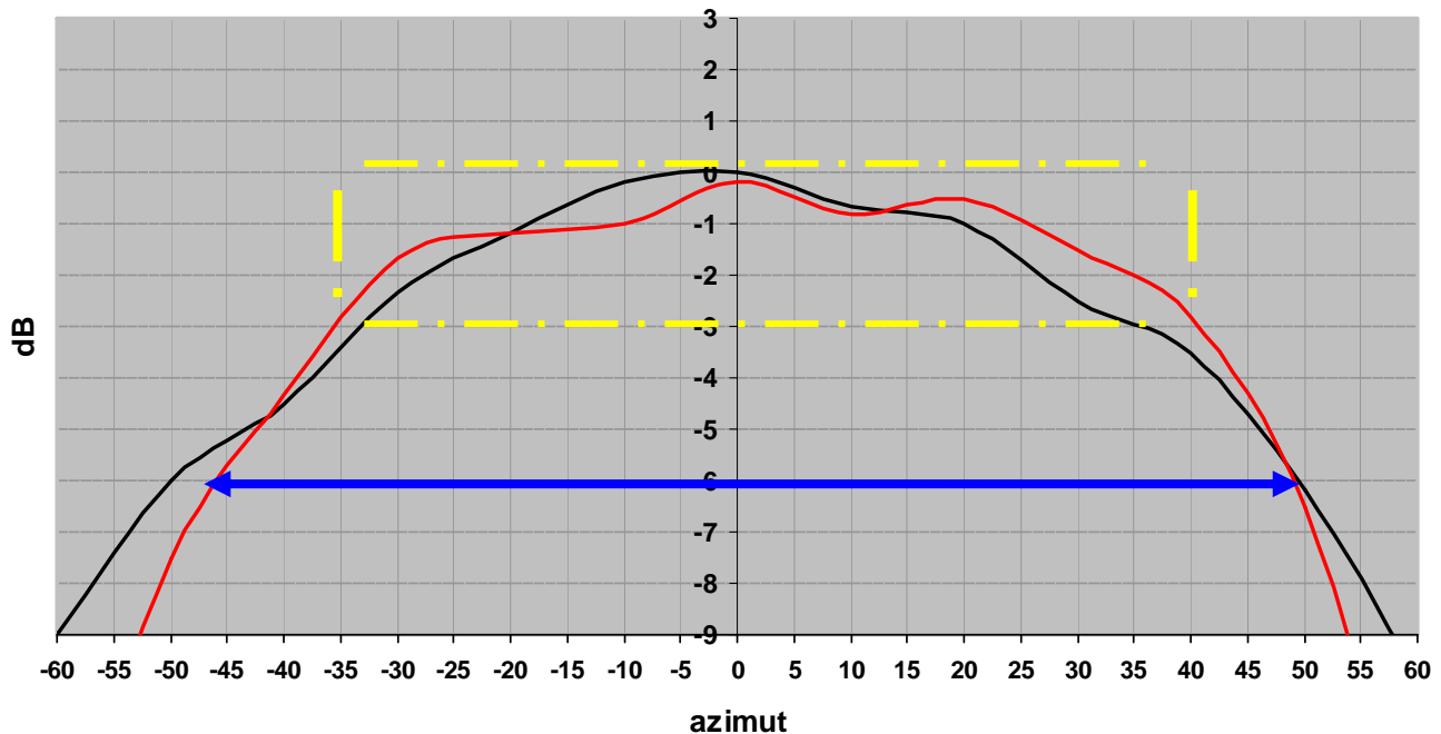
meranie hlavného vyžarovacieho laloku
