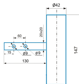
rozmery dielu MK130G
