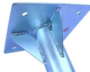
detail príruby
