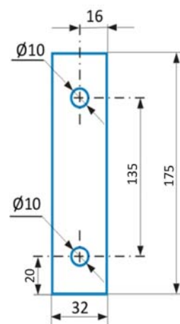
príruba
