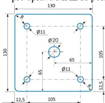
príruha KS-M R = 5mm
